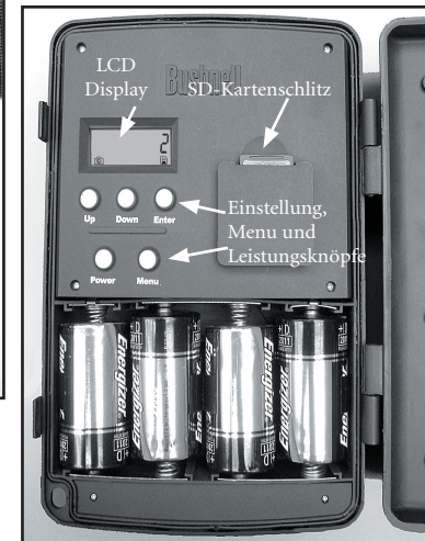
Detail Knopf und Display
