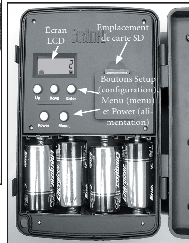
Détail des boutons et de l'écran
