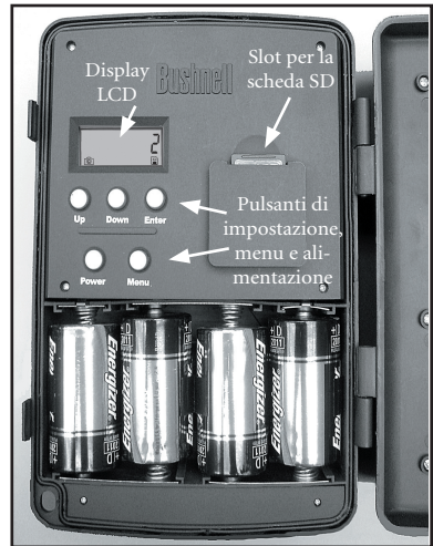
Dettaglio Pulsanti e Display
