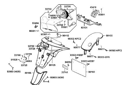
F18 後燈●後土除 Rear Light●Rear Fender -103-
