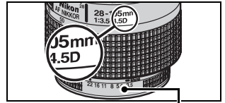
D-Nikkor Blendenring
