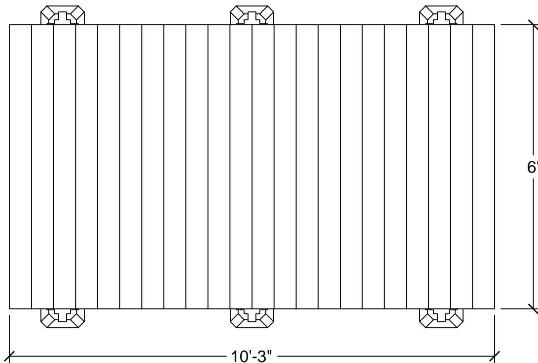
2 DECKING PLAN SCALE: 1/2" = 1' - 0"
