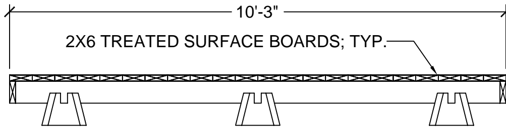
1 DECKING SECTION SCALE: 1/2" = 1' - 0"
